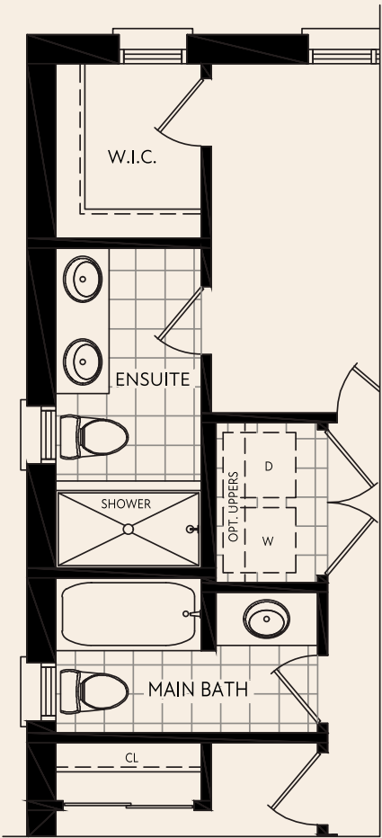
OPT. ENSUITE LAYOUT
